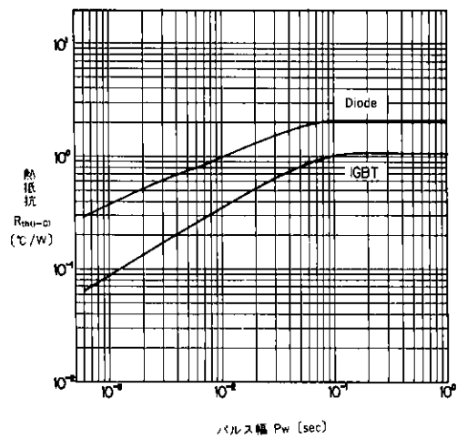
過渡熱抵抗特性 Transient Thermal Resistance
