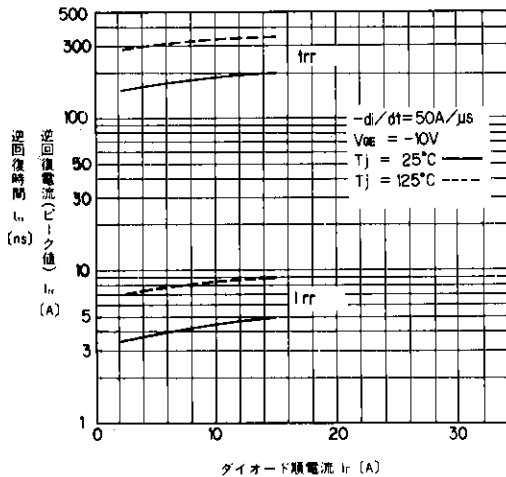
T_{rr} , I_{rr} - I_f 特性 T_{rr} , I_{rr} - I_f
